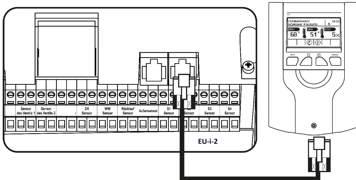
Beispielhaftes Anschließen des Zusatzventils mit dem Hauptsteuergerät EU-i-2
