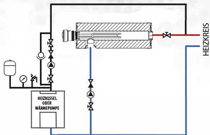
Beispielschema der Installation von MDC Nachheizmodul in einer geschlossenen Zentralheizungsanlage.
