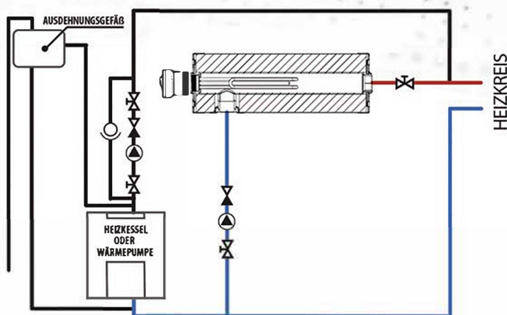
Beispielschema der Installation von MDC Nachheizmodul in einer offenen Zentralheizungsanlage.
